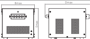
图1 JMB-25~1000外形尺寸示意图
