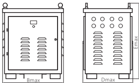
图4 JMB-6k~20k外形尺寸示意图
