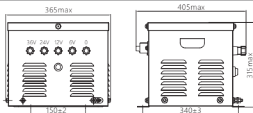
图3 JMB-5000外形尺寸示意图
