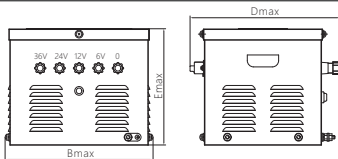
图2 JMB-1500~3000外形及安装尺寸示意图
